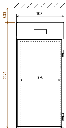
Front aanzicht
